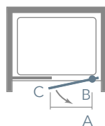
A: Door Opening B: Door Swing C: Inline Panel
